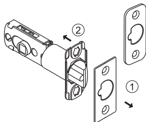
Verrou à enfoncement Drive-In Latch
